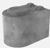
Blok D0-2 120x80x80 cm 1 550 kg 3 850 Kč
