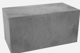
Blok RD1 160x80x80 cm 2 300 kg 4 250 Kč
